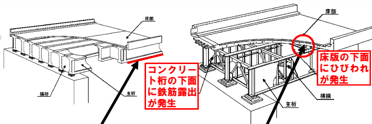
主桁の損傷（鉄筋露出）
